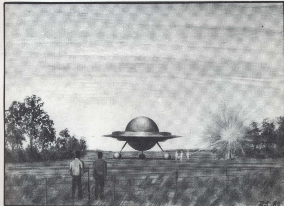
Då de passerade ett jacarandaträd riktade den av männen, som bar på detektor, ett rörligande föremål mot detta, varvid en eldstråle sköt ut och fullständigt förbrände trädet.
