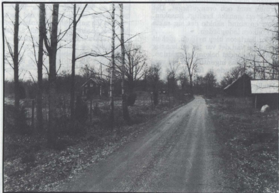
Trakten kring Norra Kväll i Småland tycks vara flitigt besökt av UFO:s. Här, vid familjen Karlssons gård, uppenbarade sig ett mystiskt "himlalus". Likt en artificiell måne sänkte sig UFO:t ner över gården och höll på kuppen på att skrämman livet av gårdens höns!
