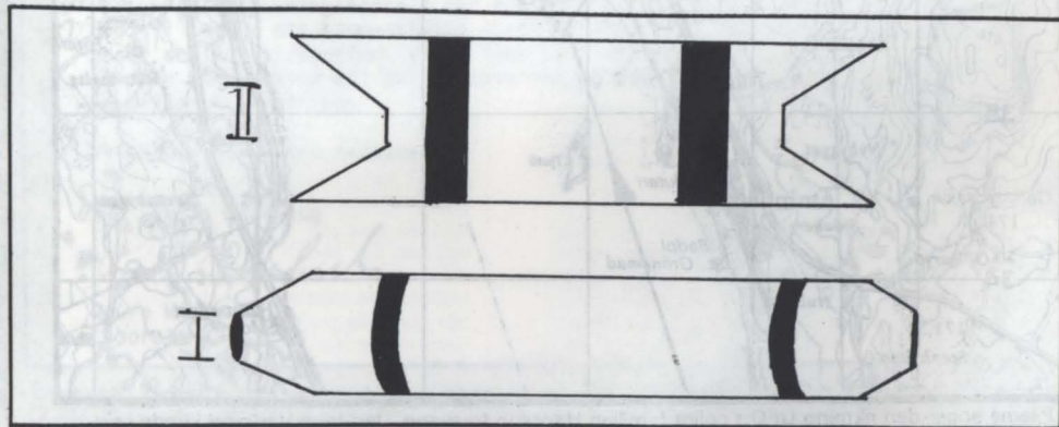
UFO:t över Vidöstern som två var för sig skilda vittnen upplevt det. Den övre skissen som observatören i Tännö såg det — den under som familjen Hansson upplevde det.
